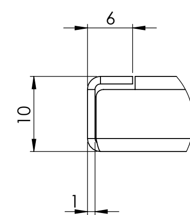
DETAIL D MĚŘITKO 2 : 1
