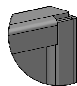
DETAIL F MĚŘITKO 2 : 1
