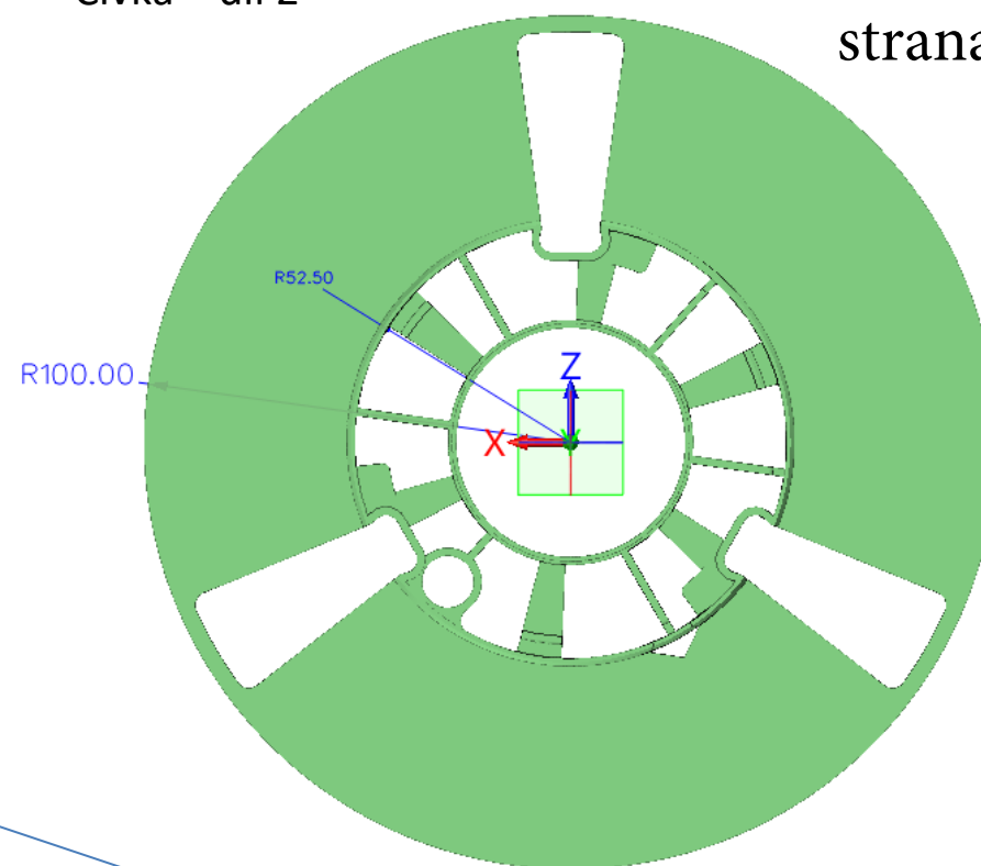
Cívka – díl 2 Hmotnost 143 g
