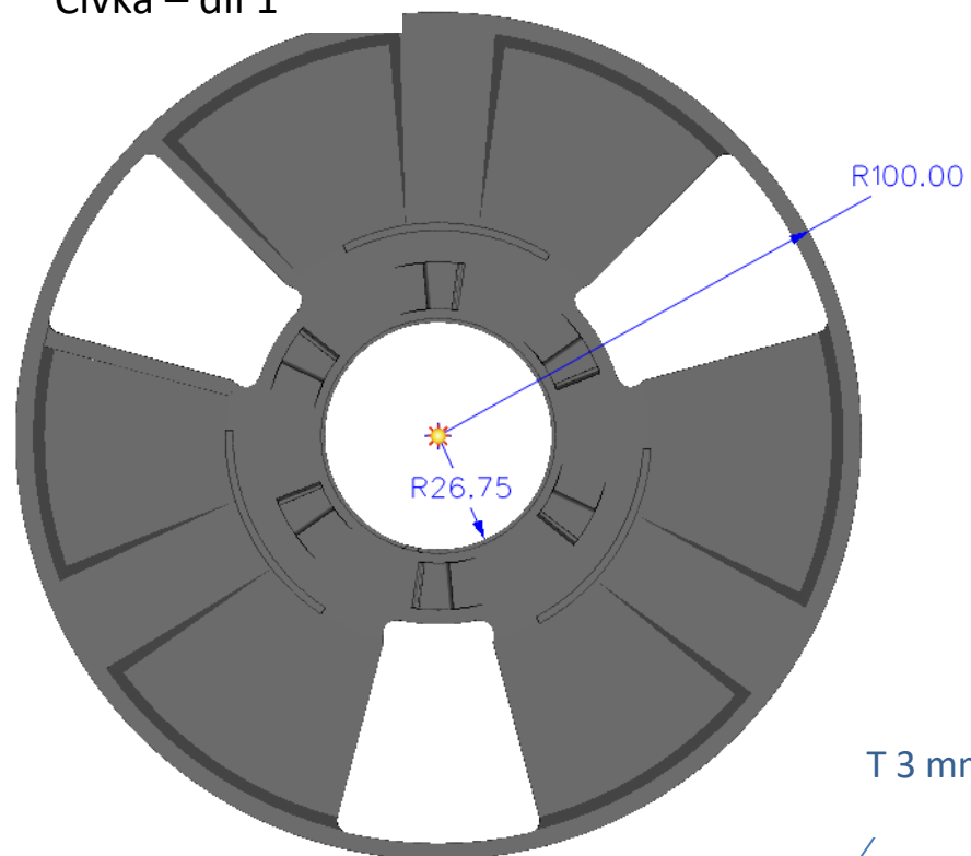
Cívka – díl 1 Hmotnost 65 g
