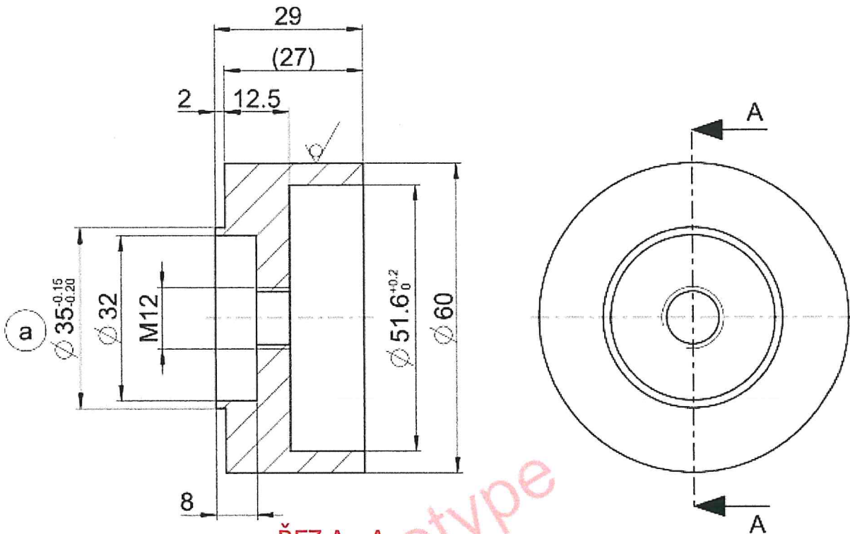
ŘEZ A - A SCHNITT A-A
